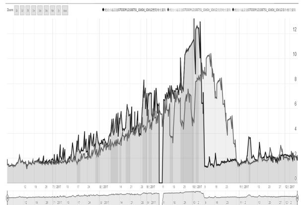
圖 15 成功小區夜間最小流量漏水預測趨勢圖
