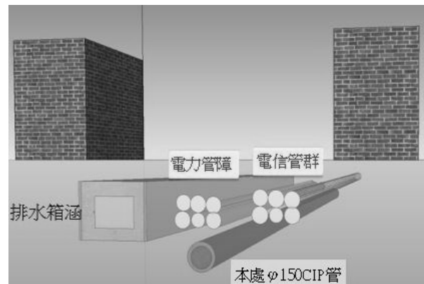
圖 9 配水管遭地下管障覆蓋示意圖
