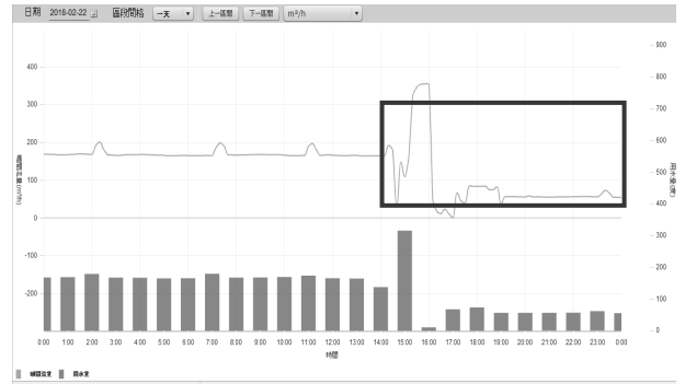
圖 18 E 系統平台顯示 A 公司 107.02.22 進水異常趨勢圖
