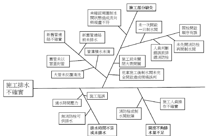
圖 2 施工排水不確實特性要因分析圖
