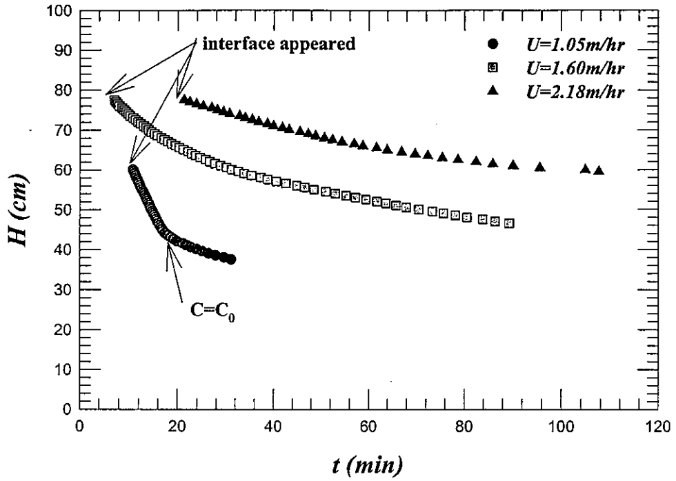
圖 6 初始濁度為 200NTU + 20 ppm as Al 之動態實驗。
