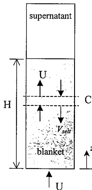
圖 1 泥毯系統模型
