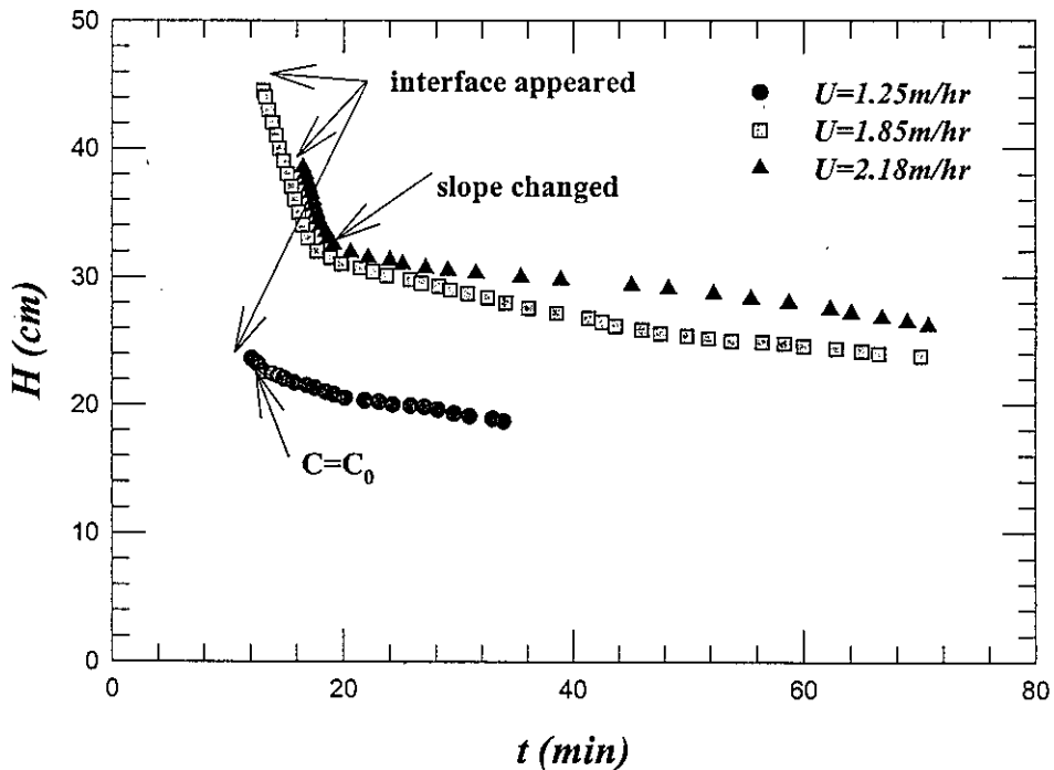
圖 5 初始濁度為 200 NTU + 12 ppm as Al 之動態實驗。
