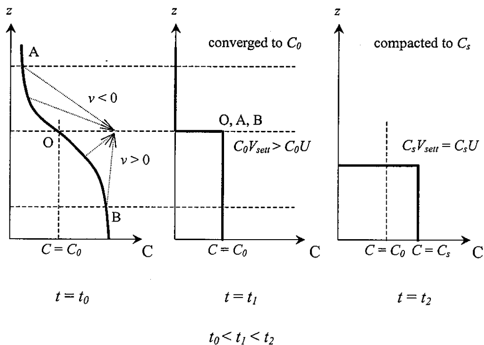
圖 3 泥毯發展過程之圖示；於 t=t_0 泥毯之最初分佈；於 t=t_1 ，泥毯在 C=C_0 收斂為均一分佈；於 t=t_2 ，泥毯自身壓密至在 C=C_s 之均一分佈。
