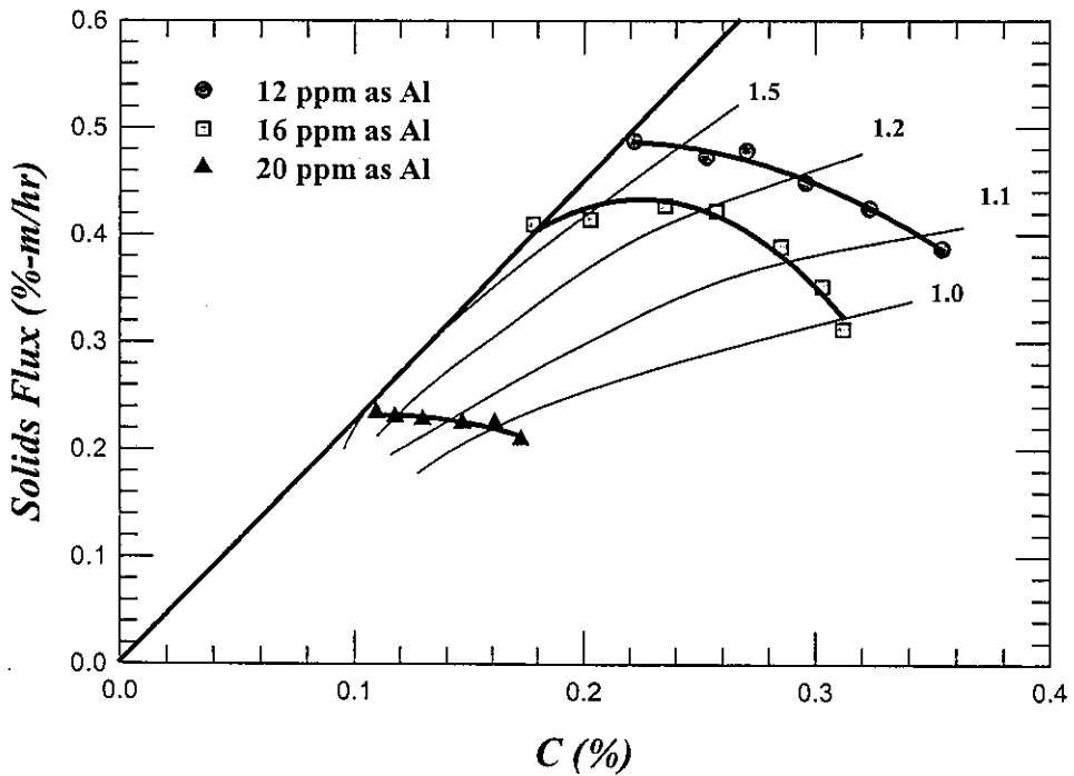
圖 7 初始濁度為 200 NTU 流化床之泥毯上浮實驗。
