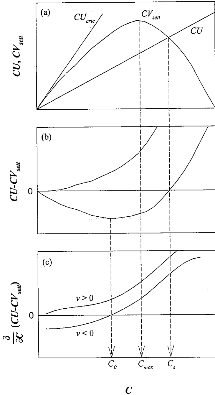
圖 2 固體通量對固體濃度之繪圖；(a) 沉降與上浮之固體通量曲線；(b) 沉降與上浮的固體通量差值；(c) 微分(b)部份，相當於系統之特性速度。
