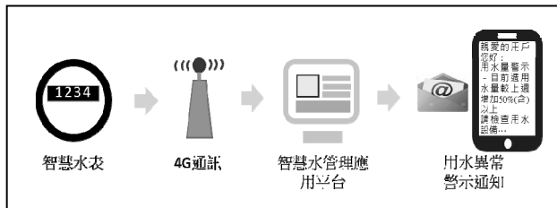
圖 1 智慧水管理系統架構
