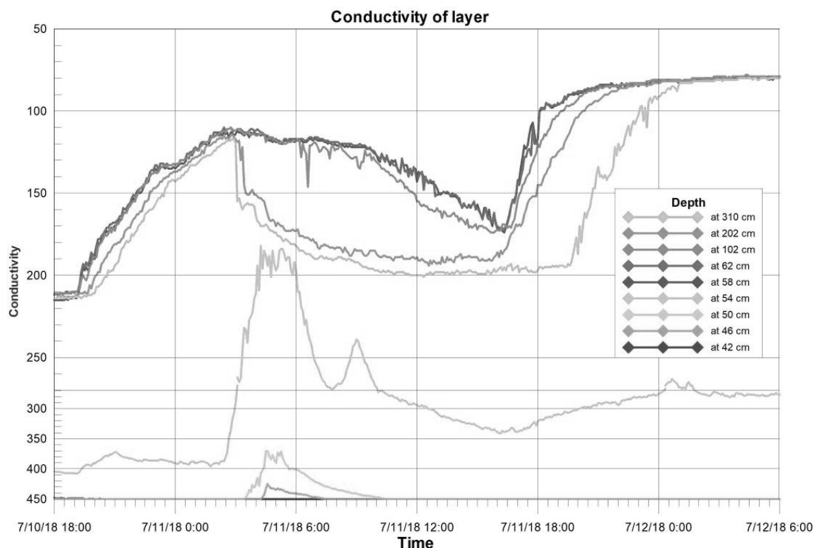
圖 7 代表層測值歷線圖 2018-07-10 18:00~07-12 06:00
