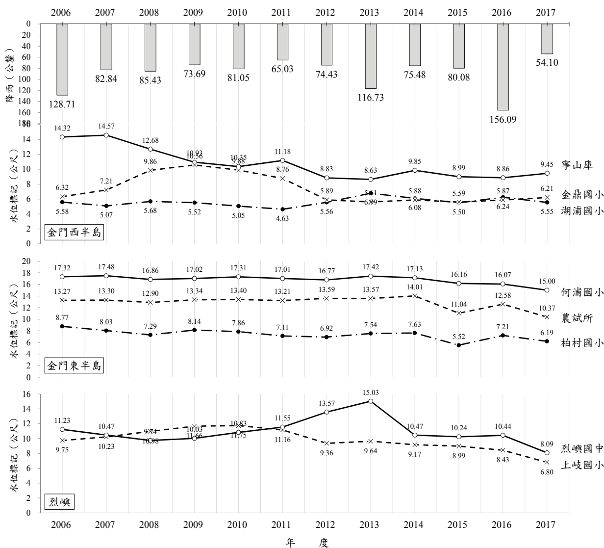
圖 6 2006~2017 年金門地區降雨及地下水位變化
