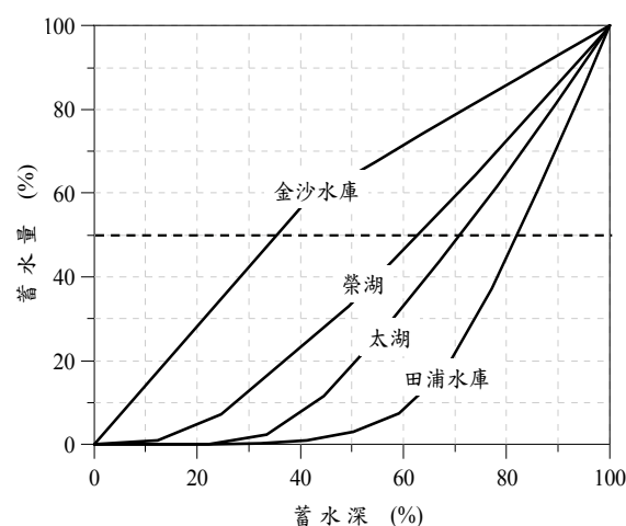
圖 4 金門主要湖庫無因次庫容曲線
