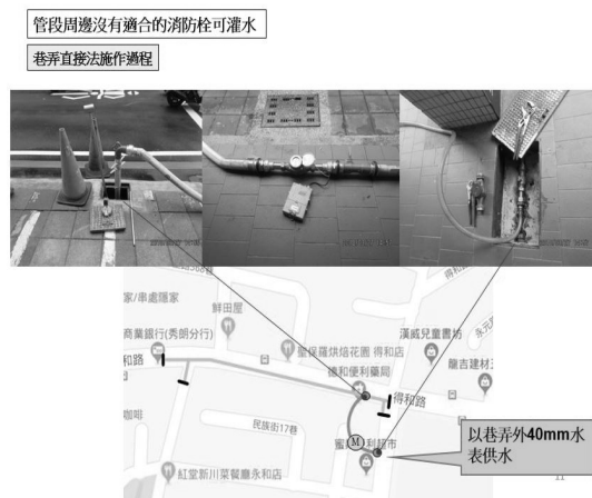
圖 15 巷弄直接法之創新作法
