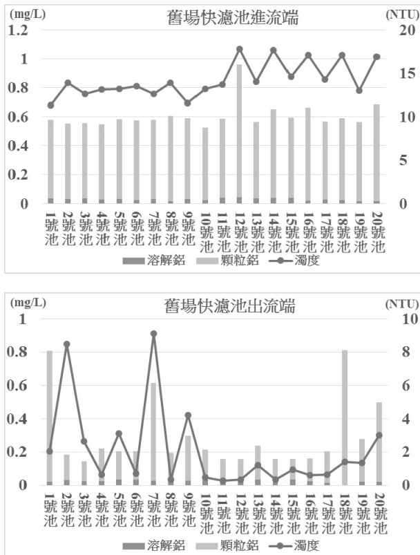
圖 7 坪頂淨水場舊場快濾池濁度及鋁
