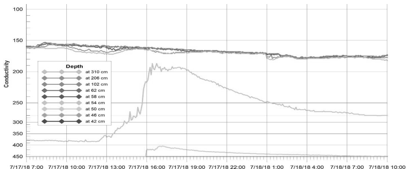
圖 9 【54cm】層測點隨時間電導度降低顯示污泥揚起
