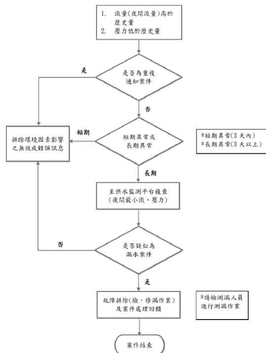
圖 3 WADA 案件接收處理流程[流量或夜間流量高於歷史量、壓力低於歷史量]
