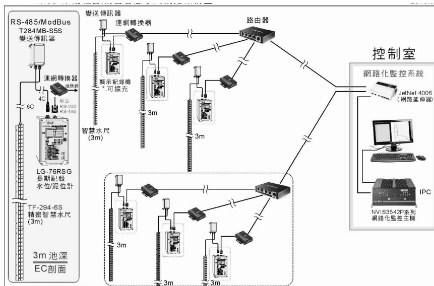
圖3 精密電導率剖面儀網路架構圖
