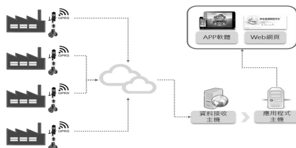
圖 14 南科應用 E 系統架構圖
