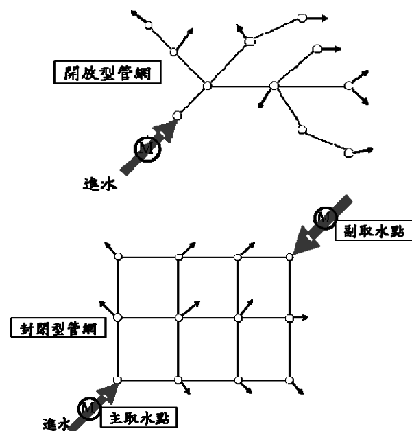
圖 1 管網形式
