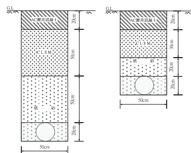
圖 1 管溝開挖標準斷面
