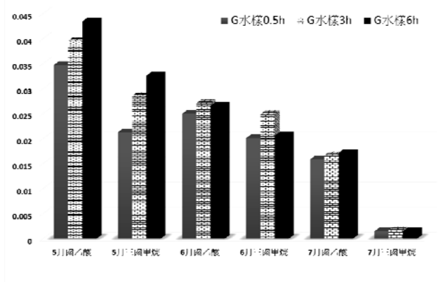
圖 12 G 水樣不同時間內 HAA5 及 THM29 變化
