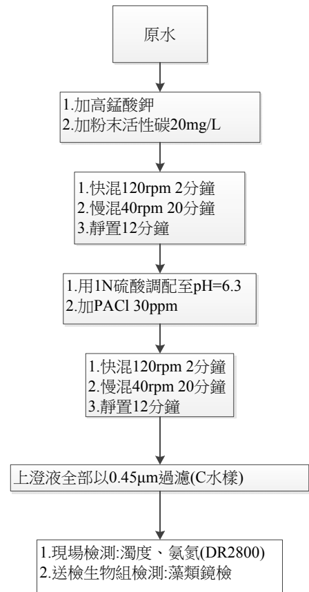
圖 3 實驗組步驟 C 流程圖
