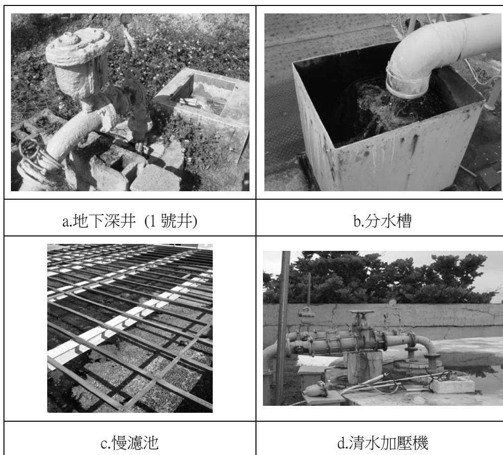
圖 2 吉貝淨水場淨水處理實況
