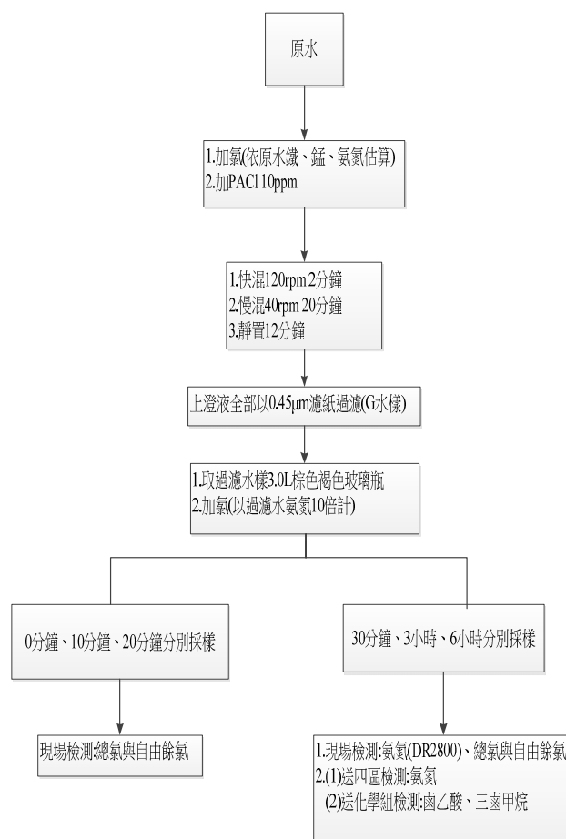
圖 7 對照組步驟 G 流程圖
