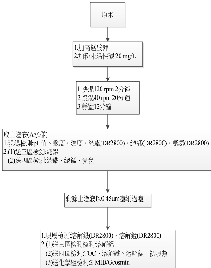
圖 1 實驗組步驟 A 流程圖
