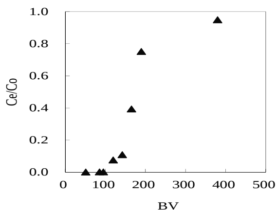
圖 9 離子交換樹脂對溴酸鹽的飽和吸附量
