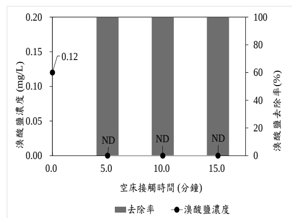
圖 10 離子交換樹脂對於淨水場水樣之空床接觸時間測試結果
