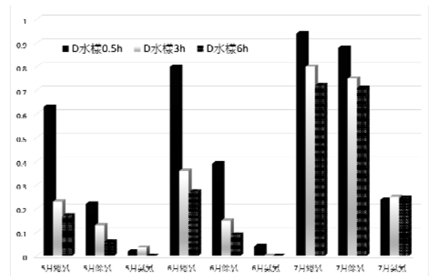
圖 13 D 水樣不同時間內總氯、餘氯及氨氮變化
