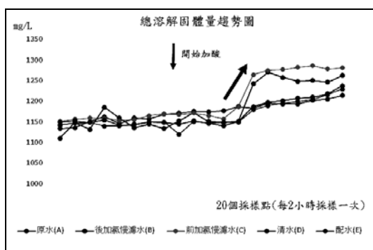
圖 6 吉貝淨水場實場驗證-總溶解固體量
