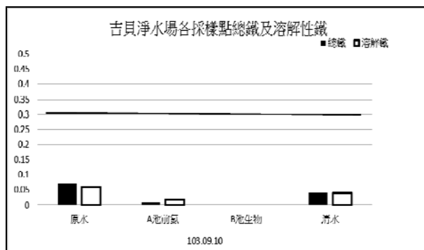
圖 15 吉貝淨水場實場驗證(第二階段)-鐵
