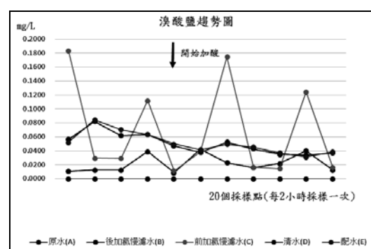
圖 8 吉貝淨水場實場驗證-溴酸鹽
