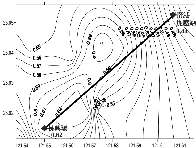
圖 9 長興場供水區自由餘氯分佈圖
