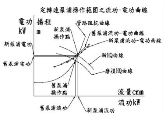
圖 10 新舊泵浦定轉速流功與電功關係
