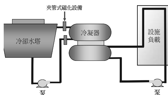
圖 3 磁化設備裝置示意
