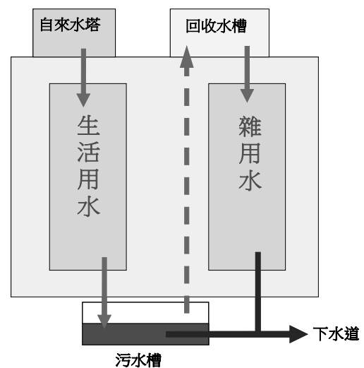
圖 7 水回收再利用示意
