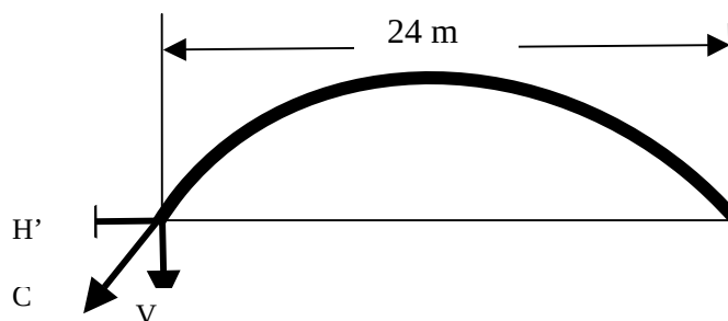
圖 2 拱頂總重分力示意
