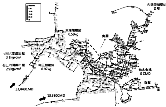
圖 5 東湖地區水理分析結果(關閉東湖路 \phi 800mm)
