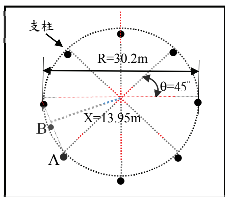
圖 3 支柱抗傾倒力矩之力臂示
