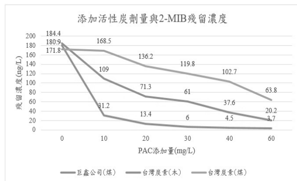
圖 2 添加活性炭劑量與 2-MIB 關係
