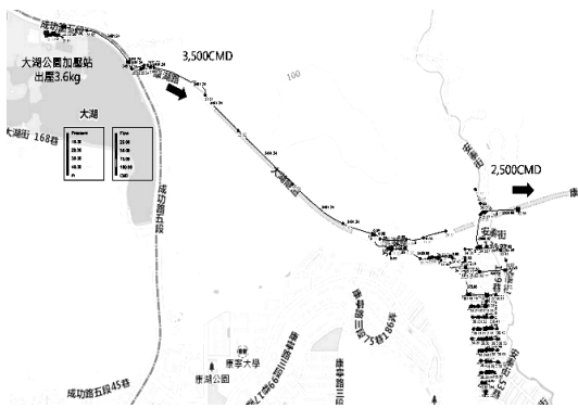
圖 6 大湖公園加壓站供水模擬
