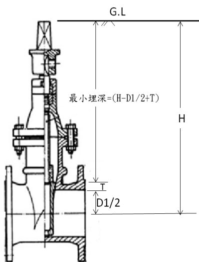
圖 1 制水閥構造
