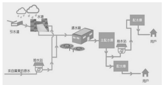
圖 1 香港飲用水供應系統示意
