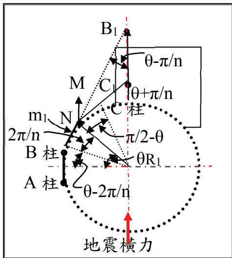
圖 5 橫撐之平面應力分析圖
