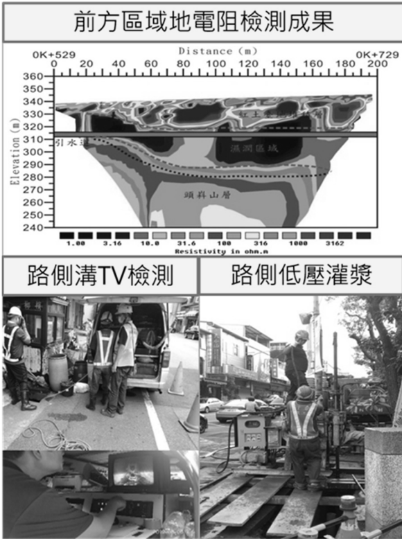
圖 11 前方探查及上方灌漿圖
