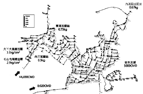
圖 4 東湖地區水理分析結果（尖峰供水、汐湖橋支援 5,000CMD）
