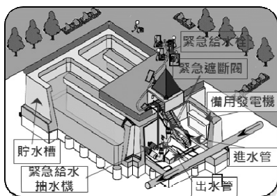
圖 1 鋼筋混凝土維生貯水槽示意圖
