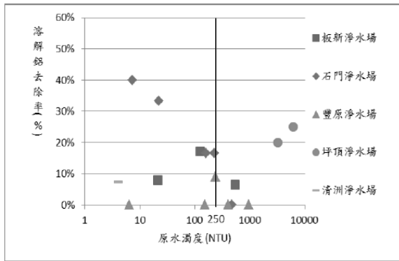
圖 3 水中殘餘溶解鋁減少百分比
