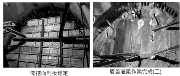
圖 10 抽坍面封板及灌漿圖
