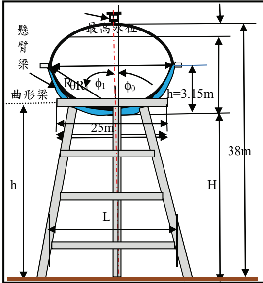
圖 2 高架水塔結構示意圖
