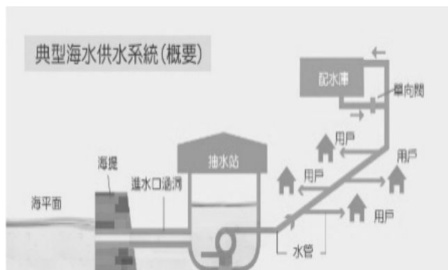
圖 2 香港海水供應系統示意
