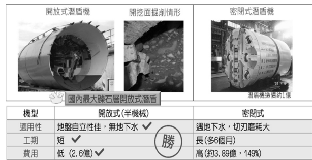
圖 4 潛盾機型式比較圖
