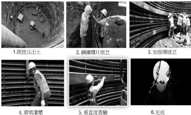
圖 6 鋼襯板施工圖
