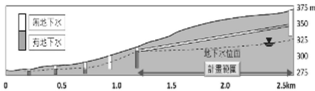
圖 2 地下水分布圖
