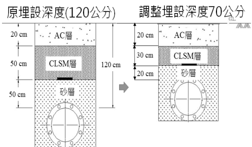
圖 4 70cm 調整後各層回填材料厚度
