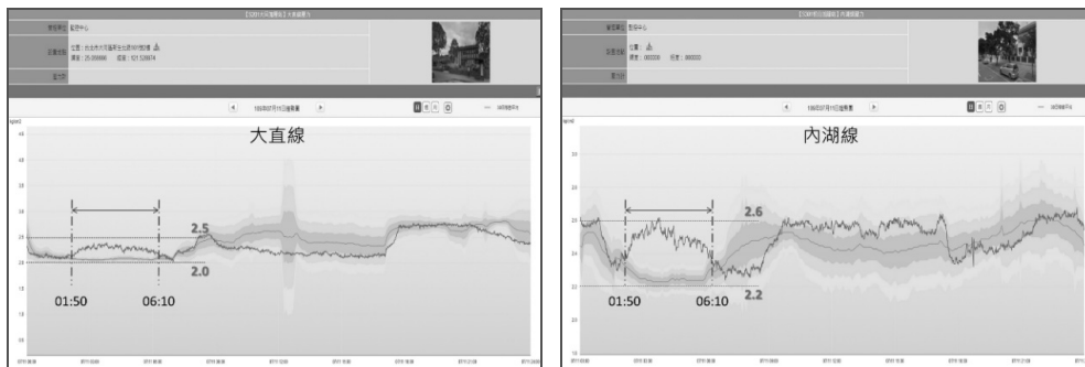
圖 15 內湖線及大直線 7 月 11 日出水壓及 30 日移動平均圖
