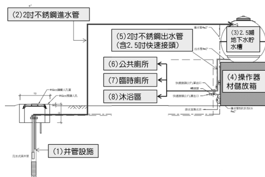
圖 5 防災地下水井示意圖
