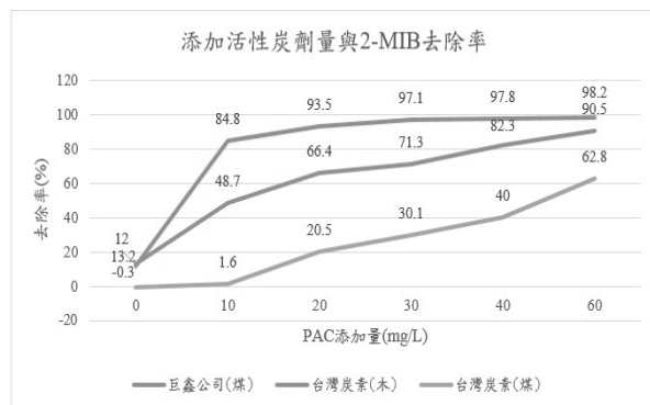
圖 1 添加活性炭劑量與 2-MIB 去除率關係
