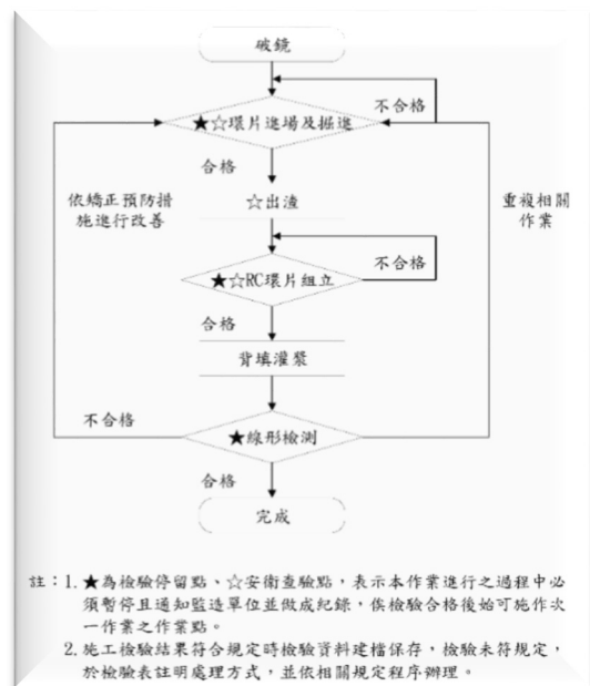
圖 8 開放式潛盾施工流程圖
