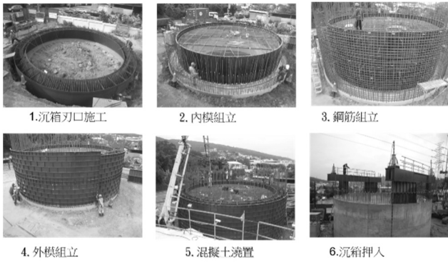
圖 5 沉箱施工步驟圖
