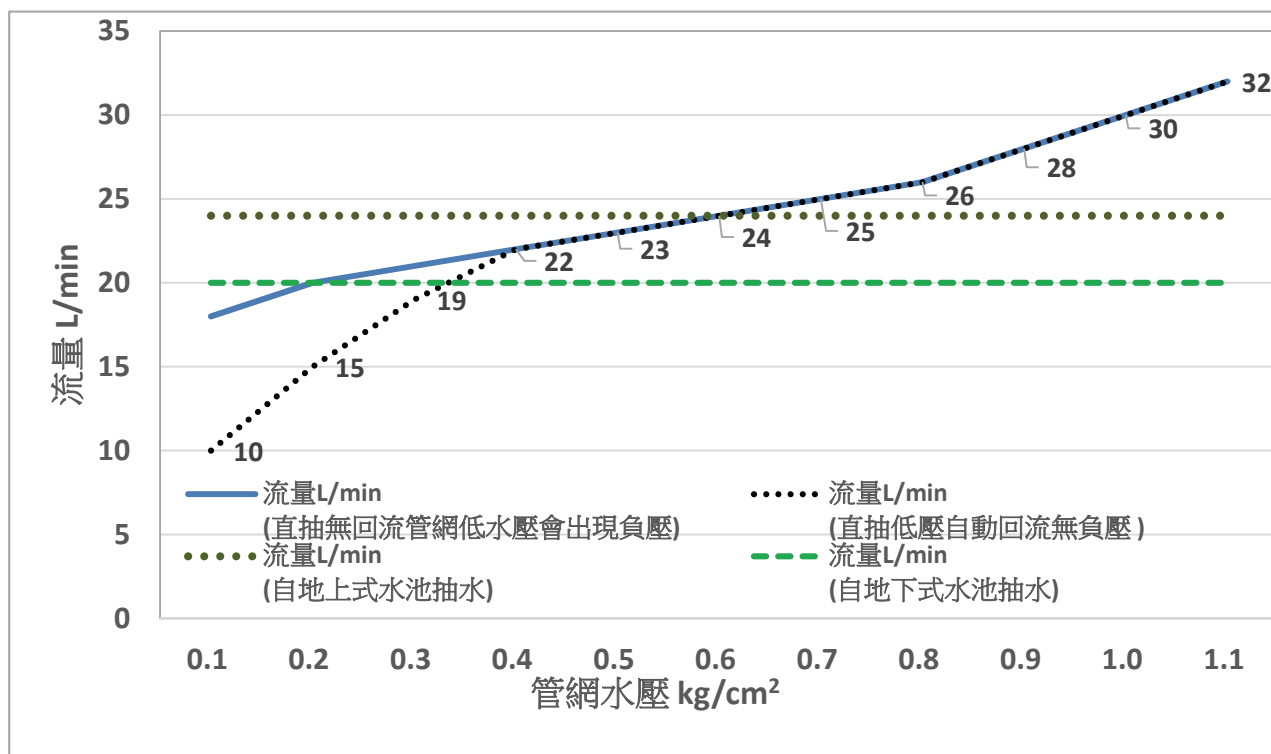
圖 5 1/2Hp 抽水機在不同情況抽水至 5 樓頂水塔的流量
