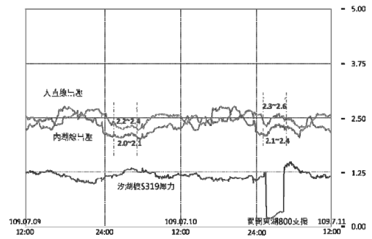
圖 14 內湖線及大直線測試前後出壓狀況
