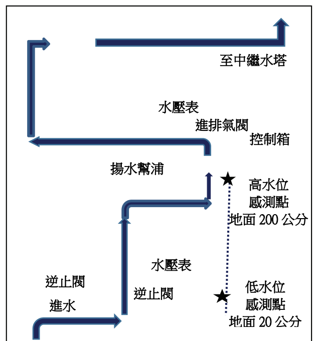
圖 1 低水壓轄區用戶直接加壓設備
