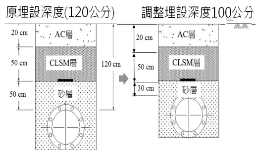
圖 5 100cm 調整後各層回填材料厚度
