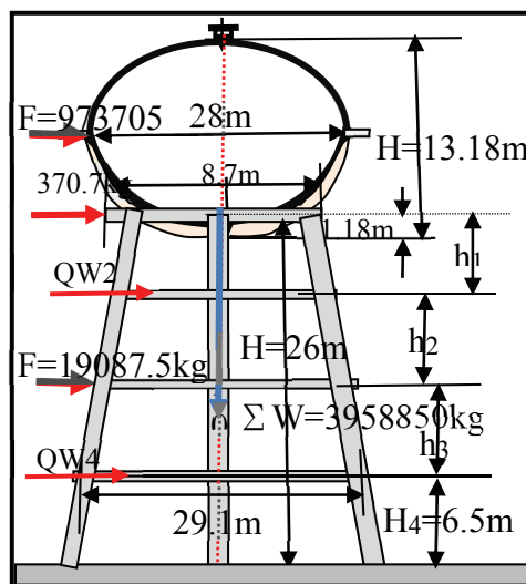
圖 4 高架水塔結構示意圖
