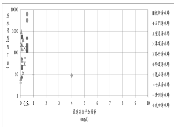
圖 1 淨水場原水濁度與最適高分子添加量關係
