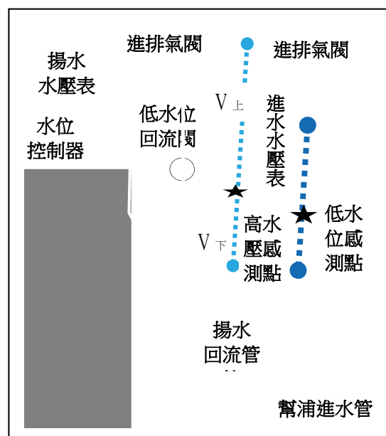
圖 4 改良式揚水設備應用實例
