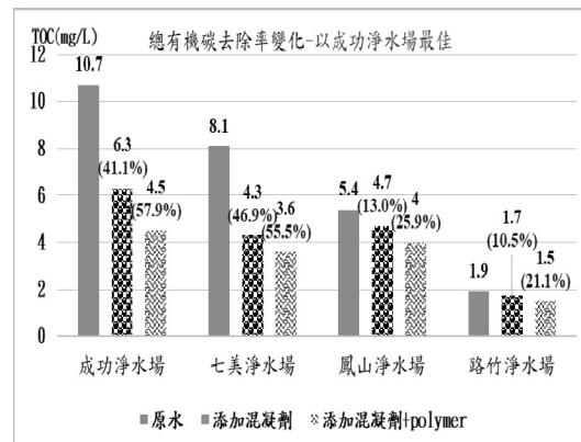
圖 6 總有機碳去除率變化(與原水比較)
