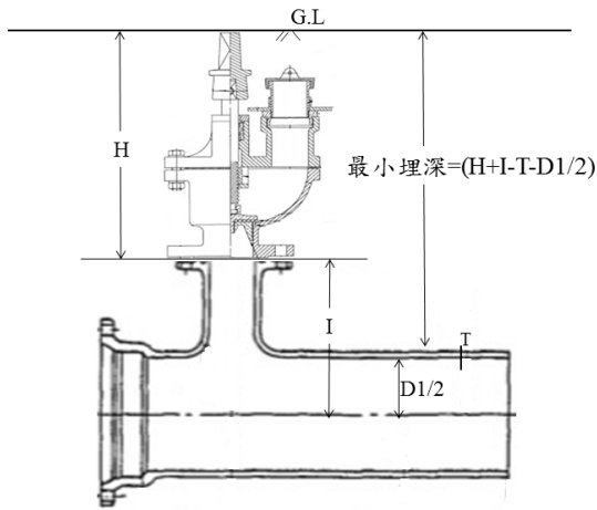
圖 2 地下式消防栓構造圖
