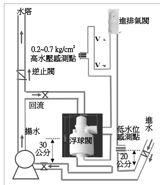
圖 2 揚水設備研發改良規劃圖說
