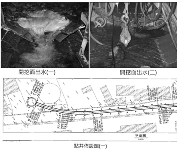
圖 12 開挖面出水及上方點井佈設圖
