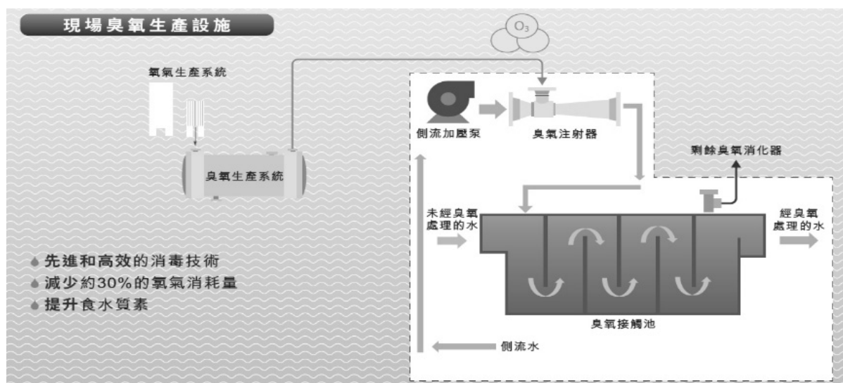
圖 7 大埔濾水廠增設現場臭氧生產設施
