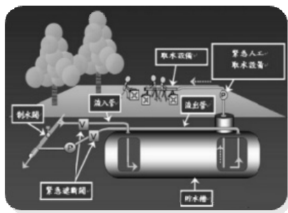
圖 2 管狀維生貯水槽示意圖
