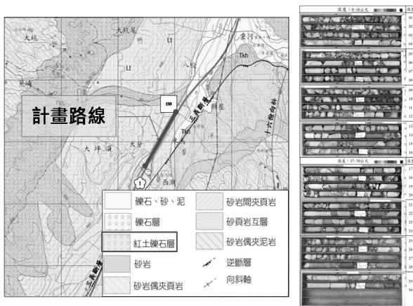
圖 3 區域岩性分布圖
