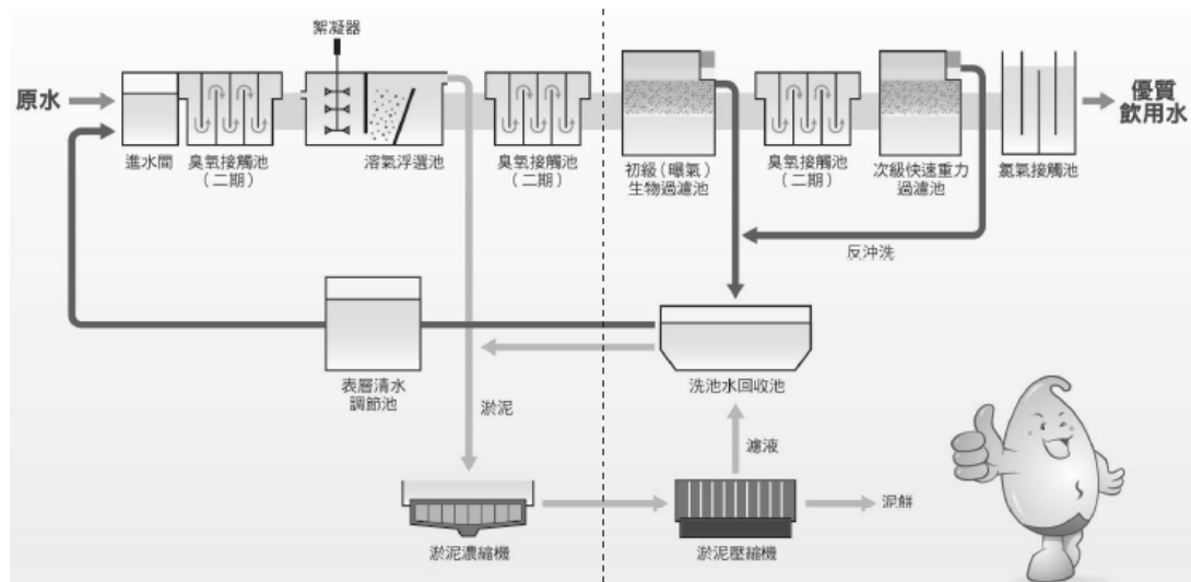
圖 9 大浦濾水廠二期擴建處理流程
