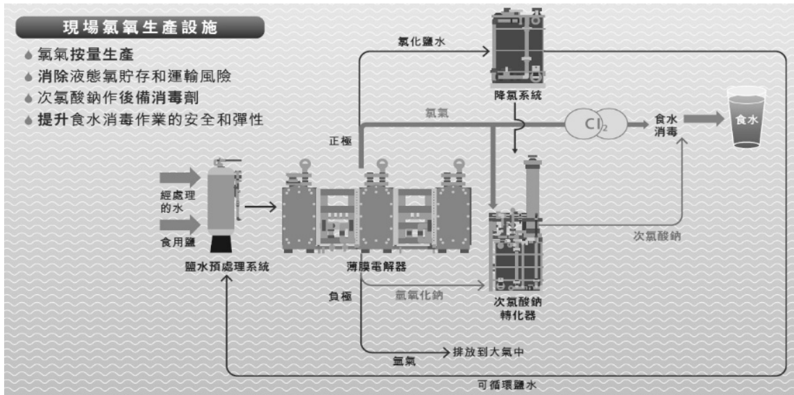
圖 8 大浦濾水廠增設現場氯消毒劑生產設施
