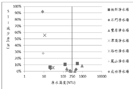
圖 4 過濾性(STI)比較
