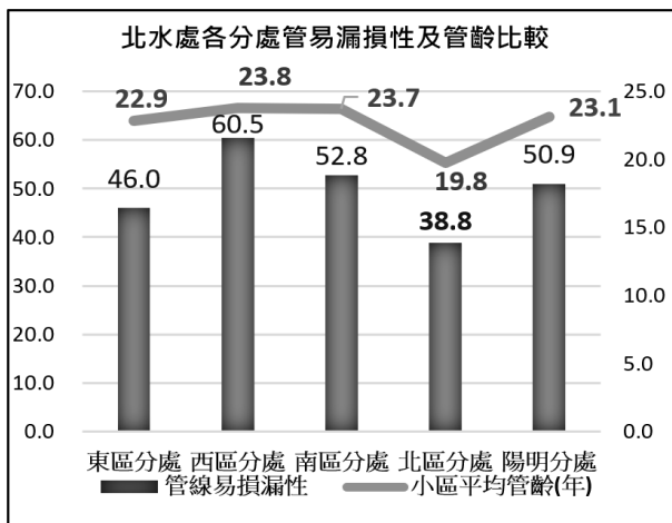
圖 3 北水處各分處管易漏損性及管齡比較圖
