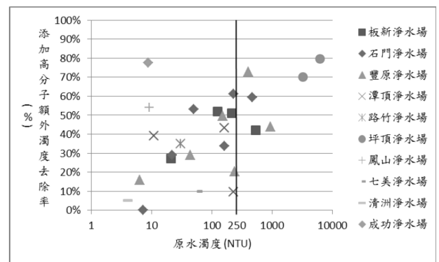
圖 2 對濁度額外去除效果
