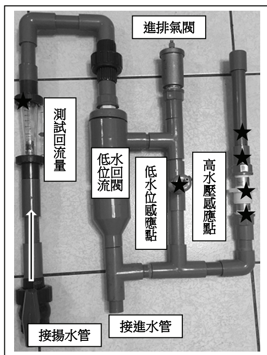
圖 3 改良式揚水測試設備零組件組裝
