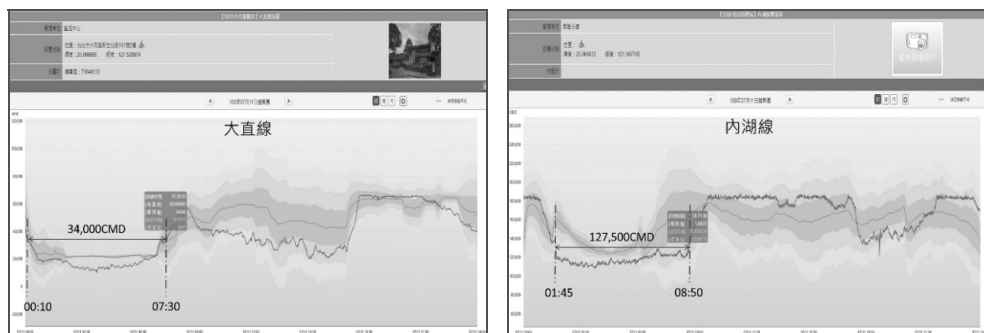
圖 16 東湖地區關閉 800mm 後實測大直線及內湖線出水量
