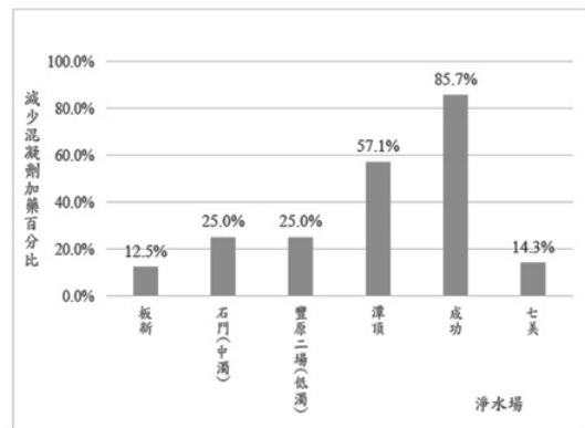
圖 5 減少混凝劑加藥量比率
