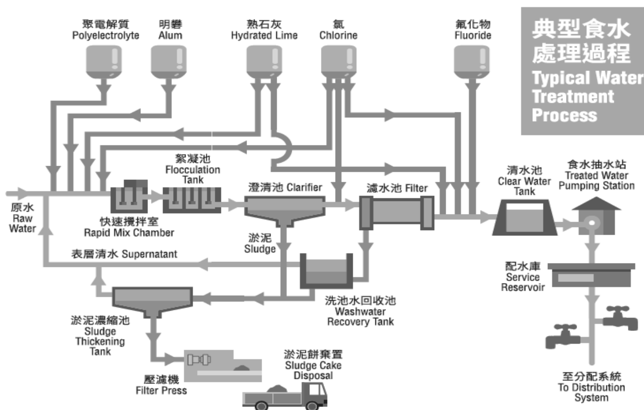
圖 4 典型香港濾水廠處理流程
