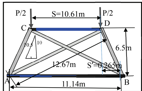
圖 6 斜撐結構示意圖
