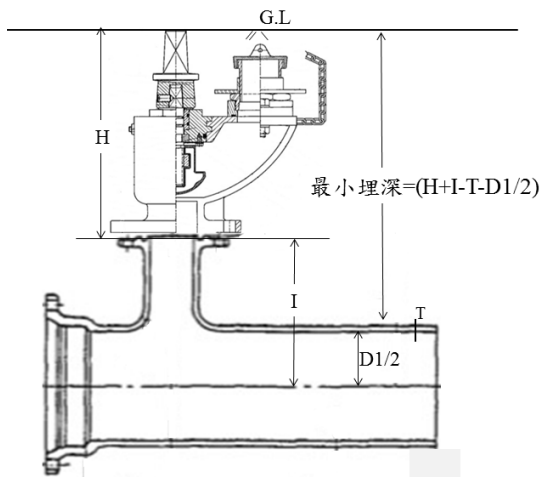
圖 3 軟密封地下式消防栓構造圖
