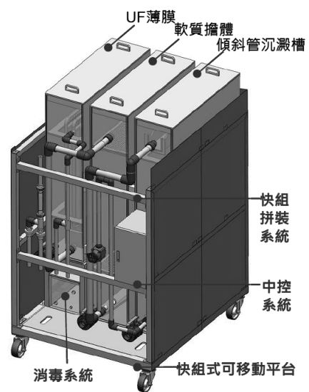
圖 18 移動式淨水設施構造圖
